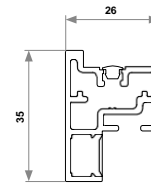
Perfil 3000 mm. frontal Lumix
