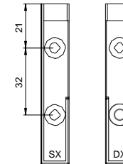
Kit sop. fijación a costado Inter
