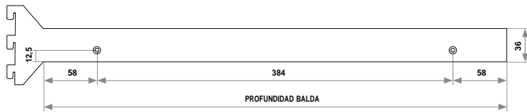
Mecanizaciones Soportes Universal
