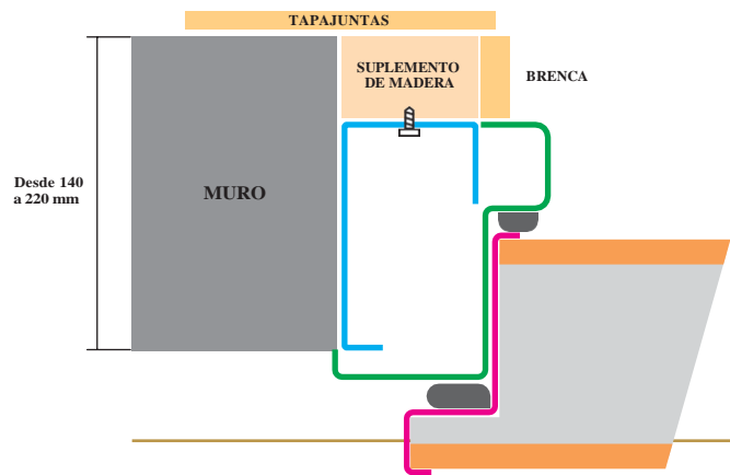
TIPO C Instalación en reforma con forro exterior
