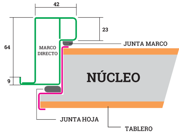
Sistema Marco Directo
