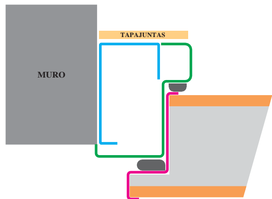
TIPO B Instalación en chalet
